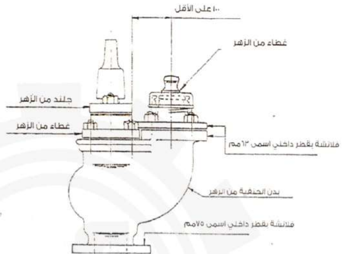
شكل استرشادي لخنقية صريق ذات محبس لولبي
